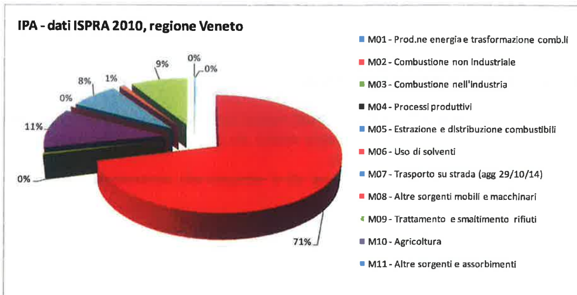
Figura 9 – Stima delle emissioni di IPA a livello regionale nel 2010 (fonte: disaggregazione provinciale dell'inventario nazionale ISPRA 1990-95-00-05-10, versione 29/10/2014).
