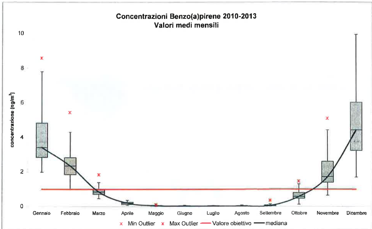
Figura 4 – Concentrazioni medie mensili di Benzo(a)pirene (2010-2013) valutate per tutte le stazioni della rete regionale di monitoraggio della qualità dell'aria situate in pianura. (Fonte: ARPAV- Osservatorio Regionale Aria).
