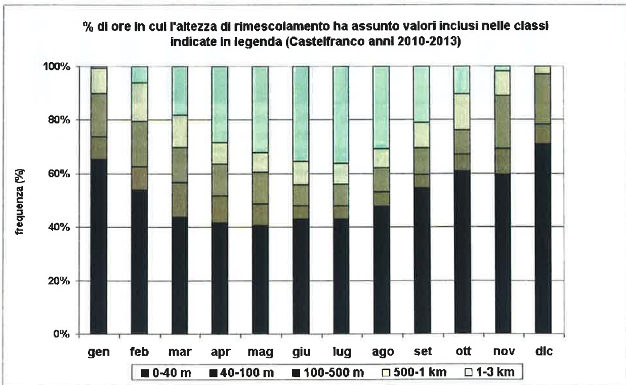
Figura 6 – Altezza dello strato di rimescolamento valutata presso la stazione di Castelfranco per gli anni 2010-2013. Suddivisione percentuale dei valori nelle classi indicate in legenda.
