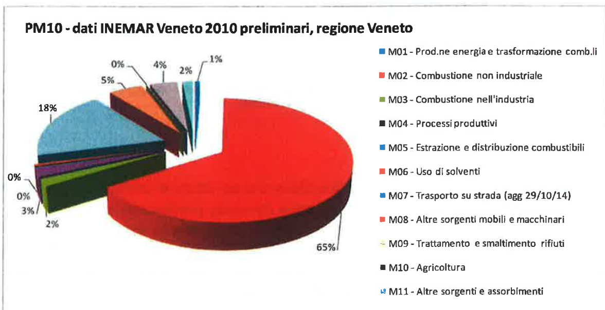
Figura 8 – Stima delle emissioni di PM10 a livello regionale nel 2010 (fonte: INEMAR Veneto 2010, versione preliminare).
